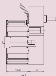
motor M42
